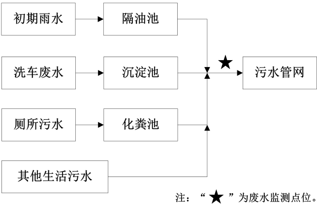
图4-1 废水处理流程图
